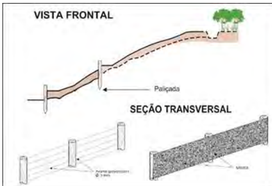
Figura 55 Esquema de retentores de sedimentos com utilização de mantas
