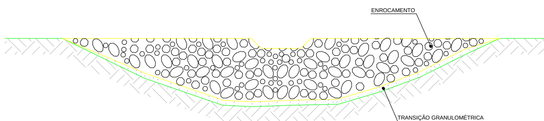
Figura 53 Exemplo de Diques implantados no Rompimento da Barragem de Fundão em Mariana – MG
