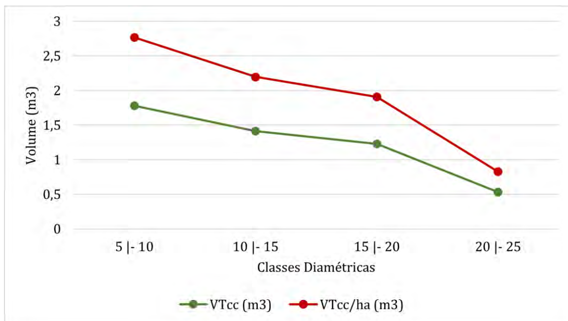
Figura 47 Volumetria (m 3 ) por Classe Diamétrica em Campo Sujo
