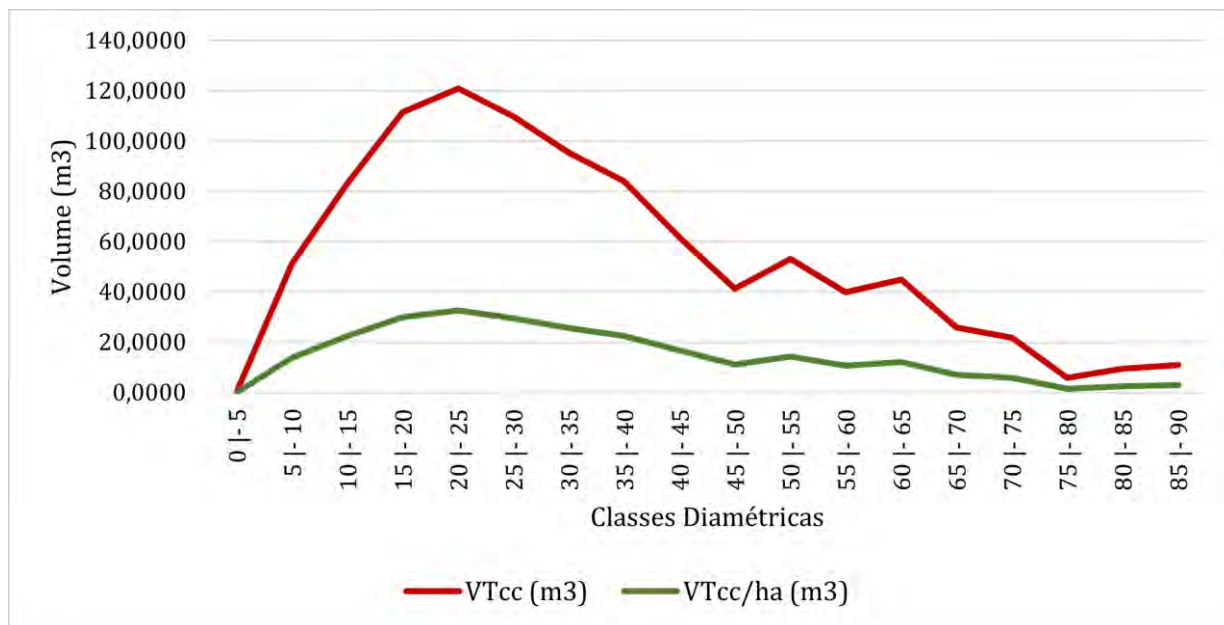
Figura 35 Volumetria (m 3 ) por Classe Diamétrica na Mata Ripária
