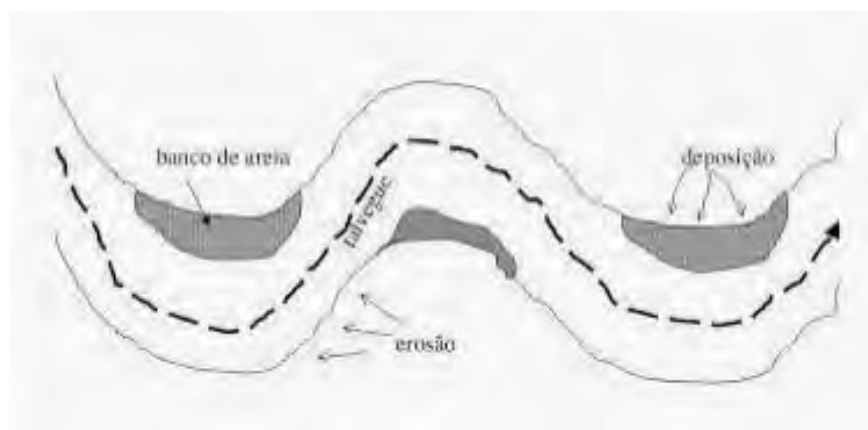
Figura 64 Modelo de sedimentação de material em cursos d'água meandriformes.
