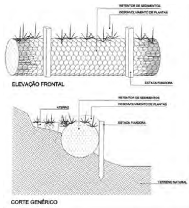
Figura 54 Esquema de retentores de sedimentos com fibra vegetal
