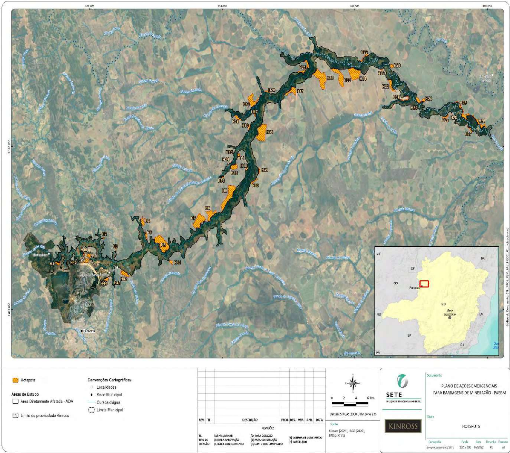
Figura 72 Localização dos Hotspots indicados para as ações de dessedentação da fauna.
