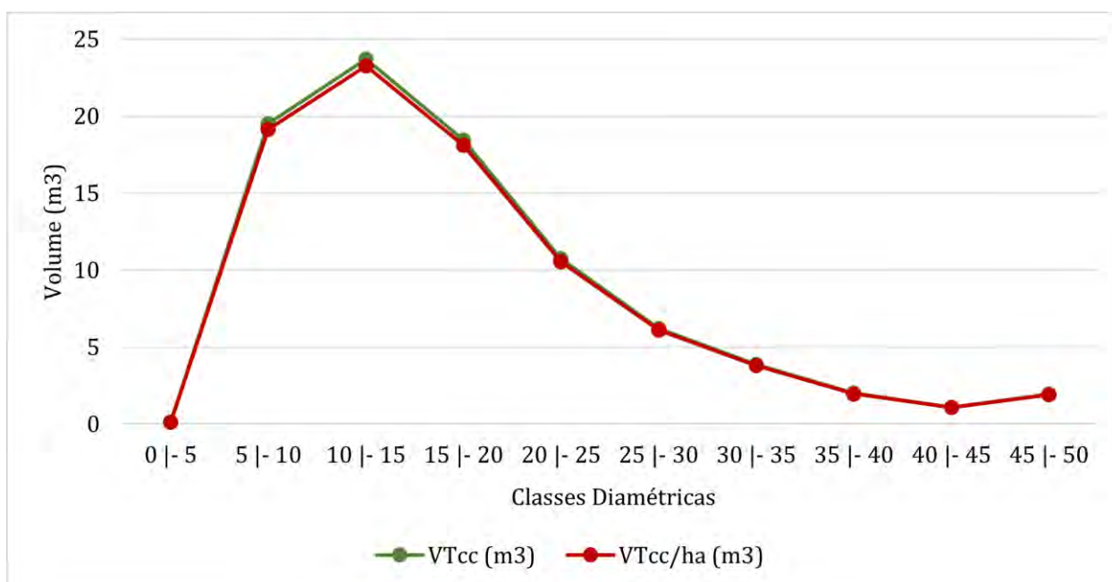
Figura 39 Volumetria ( \text{m}^3 ) por Classe Diamétrica em Cerrado Denso
