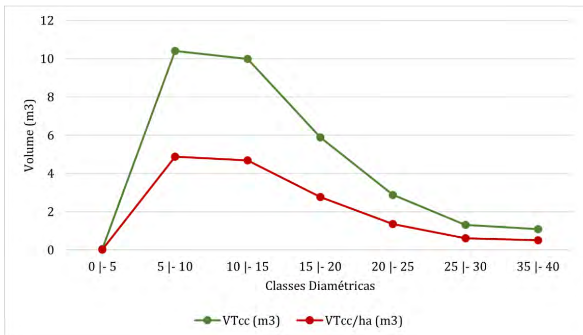
Figura 45 Volumetria ( \text{m}^3 ) por Classe Diamétrica em Cerrado Ralo em Regeneração
